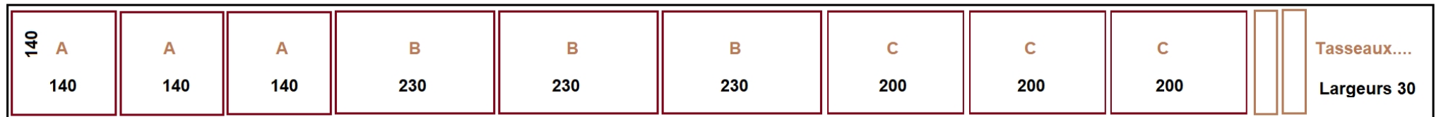
PLANCHE 2 : 18x150 Brut Longueur 2,00 m
