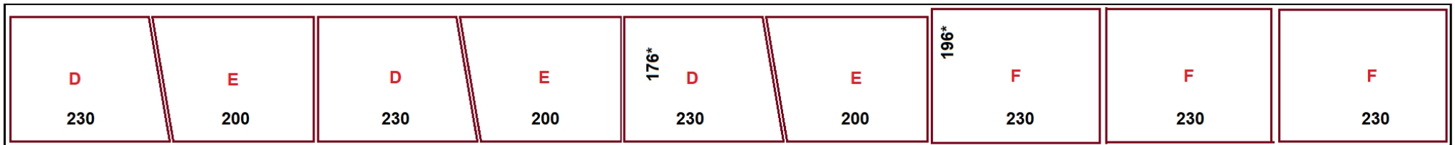
PLANCHE 1 : 18x200 Brut Longueur 2,00 m
